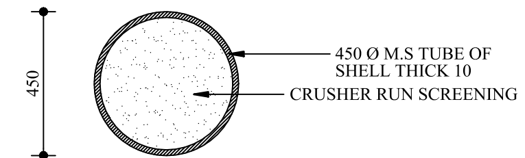
SECTION - AA (SCALE - 1 : 10)
