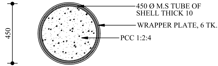
SECTION - CC (SCALE - 1 : 10)
