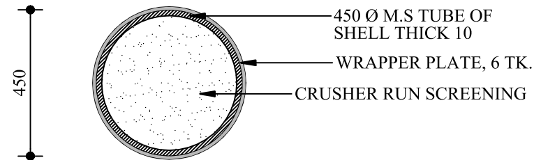
SECTION - BB (SCALE - 1 : 10)
